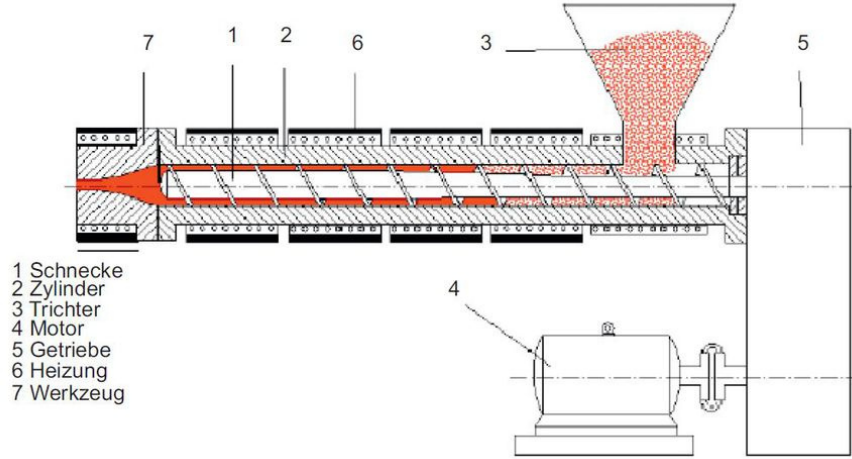
Abbildung 42: Kunststoffextruder
