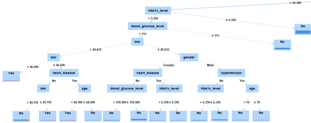
Abbildung 32: Teil des Klassifikationsbaum f_{T_2, \kappa_2}
