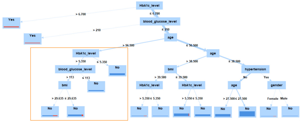
Abbildung 31: Klassifikationsbaum f_{T_1, \kappa_1} für die Diabetes-Prädiktion
