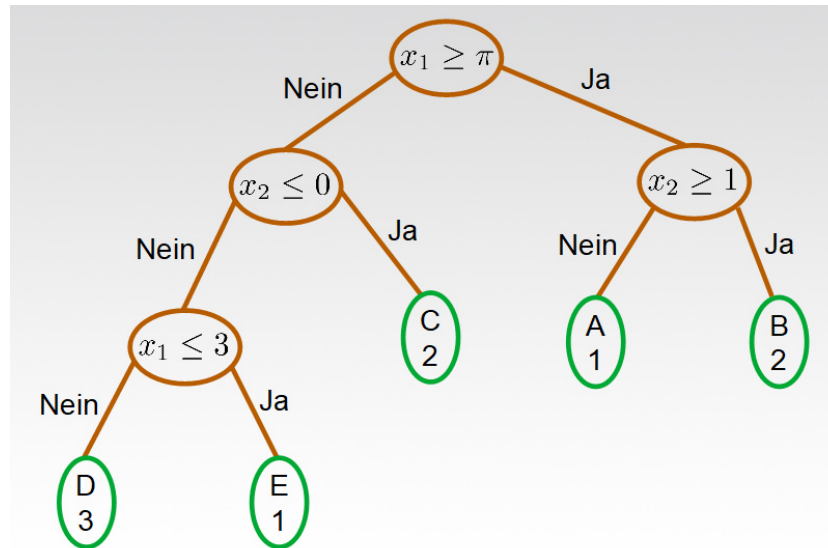
Abbildung 29: Baumartiger Klassifikator
