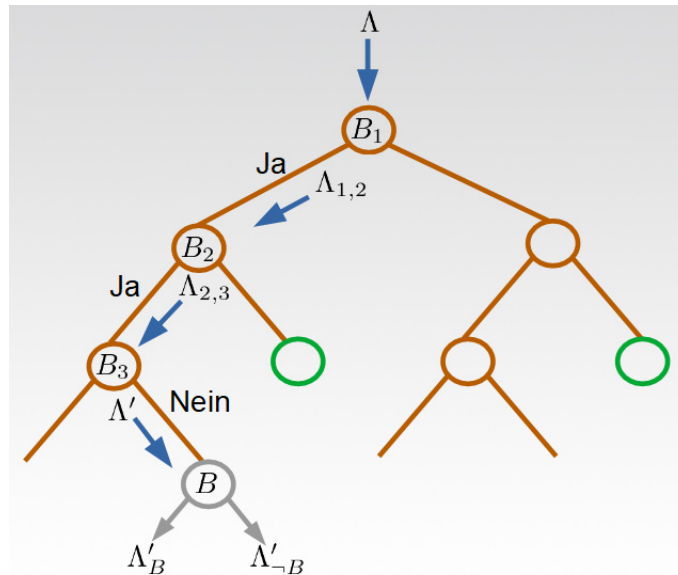
Abbildung 30: Rekursive Erzeugung eines Klassifikationsbaums
