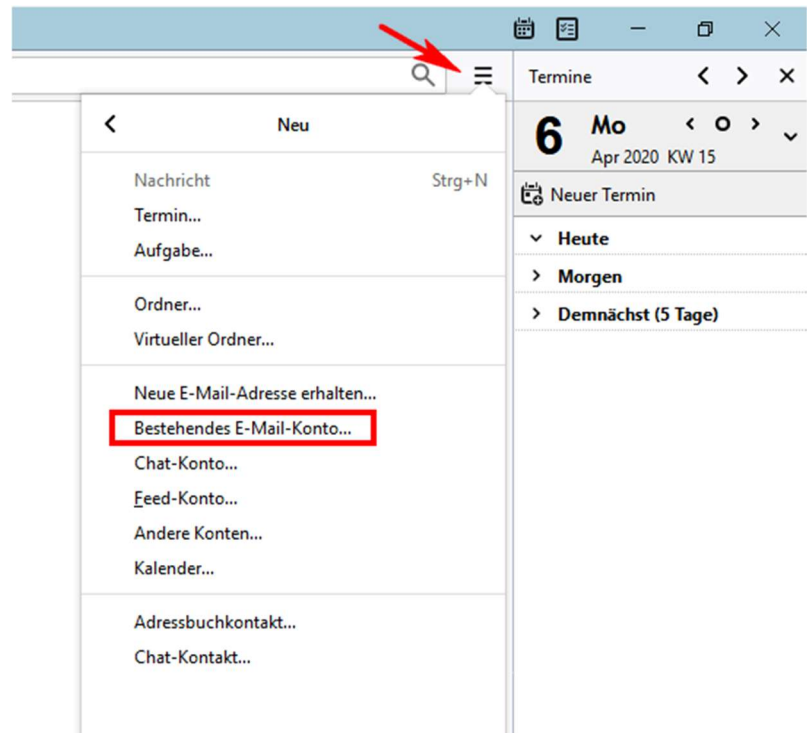
Abbildung 1: Konfigurationseinstellungen öffnen
